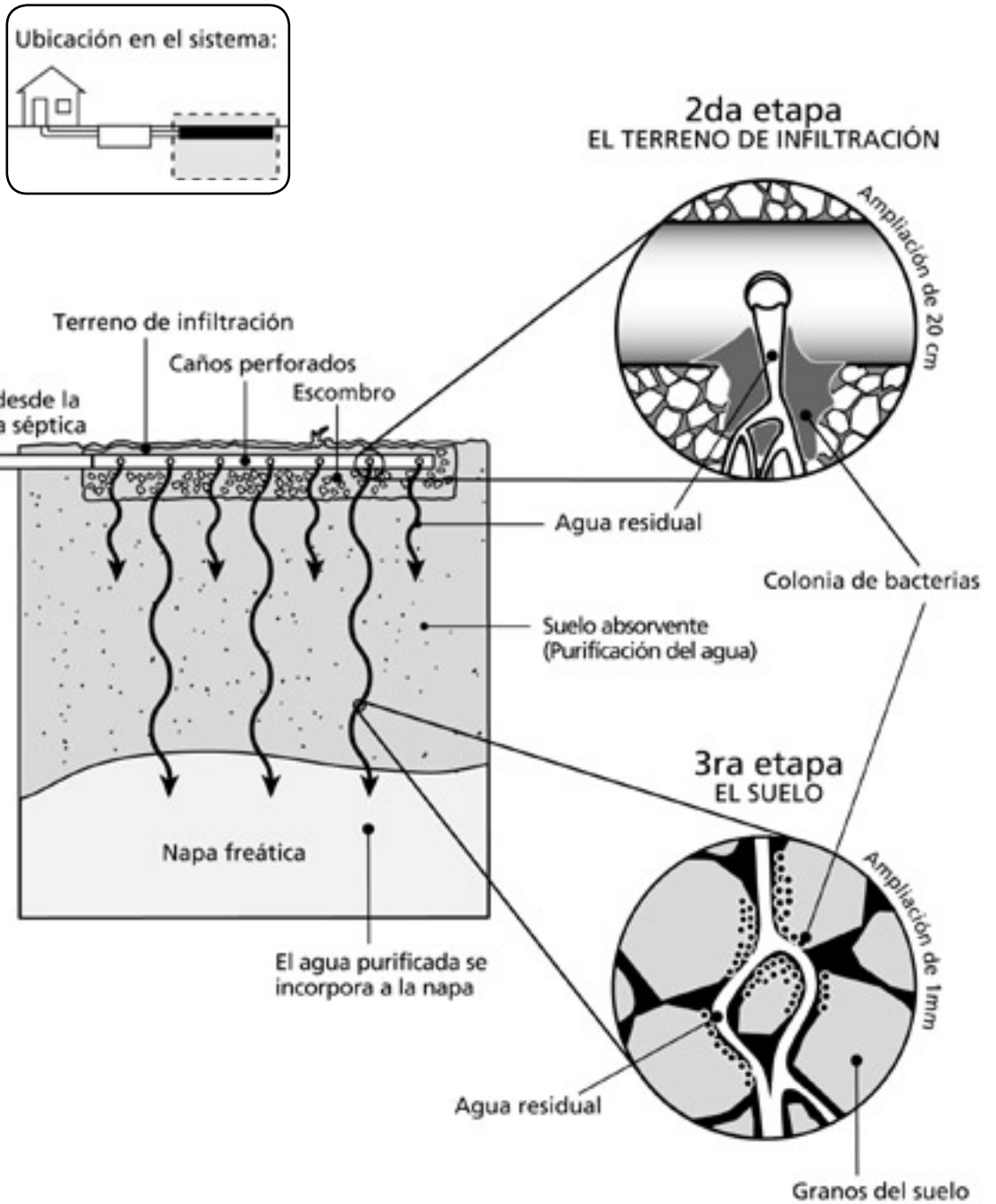
FIGURA 4 - CÓMO FUNCIONAN EL TERRENO DE INFILTRACIÓN Y EL SUELO - 2º y 3º Etapas
